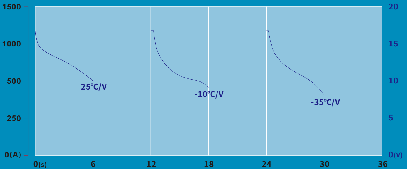
▲ TSWB-LP12V100AH在不同温度环境下的脉冲放电特性 TSWB-LP12V100AH IMPULSE DISCHARGE AT DIFFERENT TEMPERATURE
